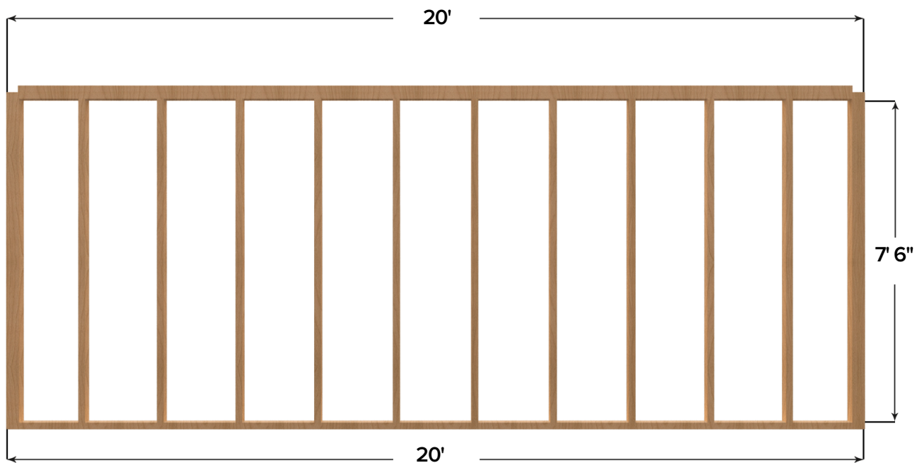
LEFT WALL
